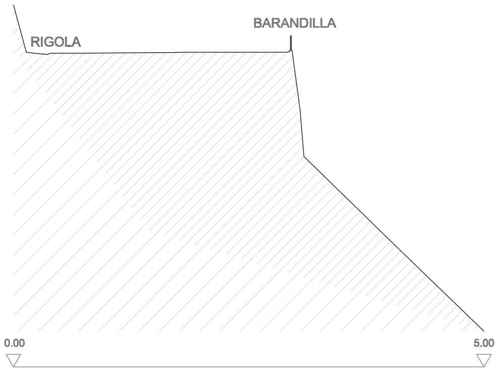
SECCIÓ D-D' 1: 250
