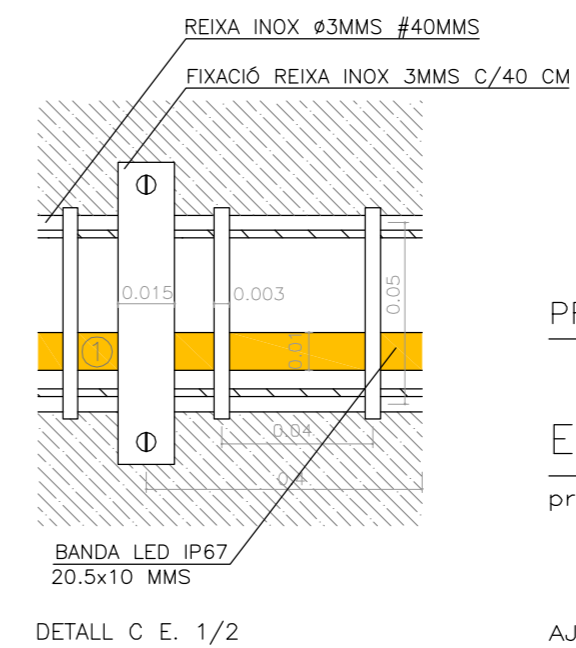
DETALL C E. 1/2
