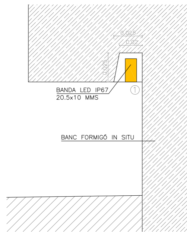
DETALL A E. 1/2
