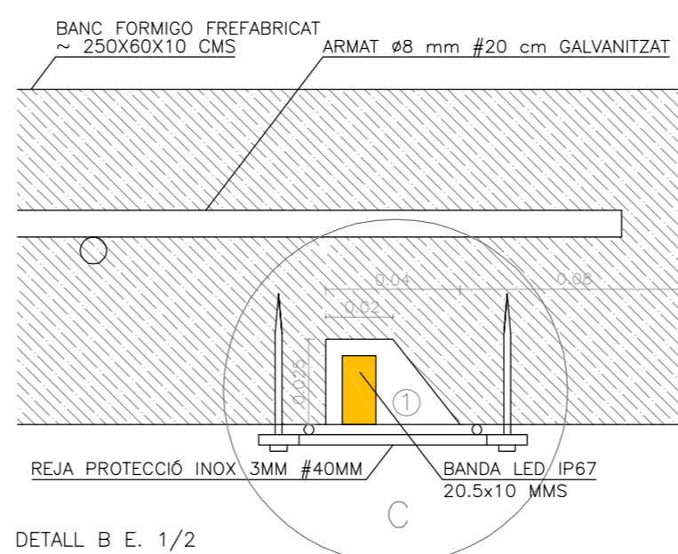
DETALL B E. 1/2
