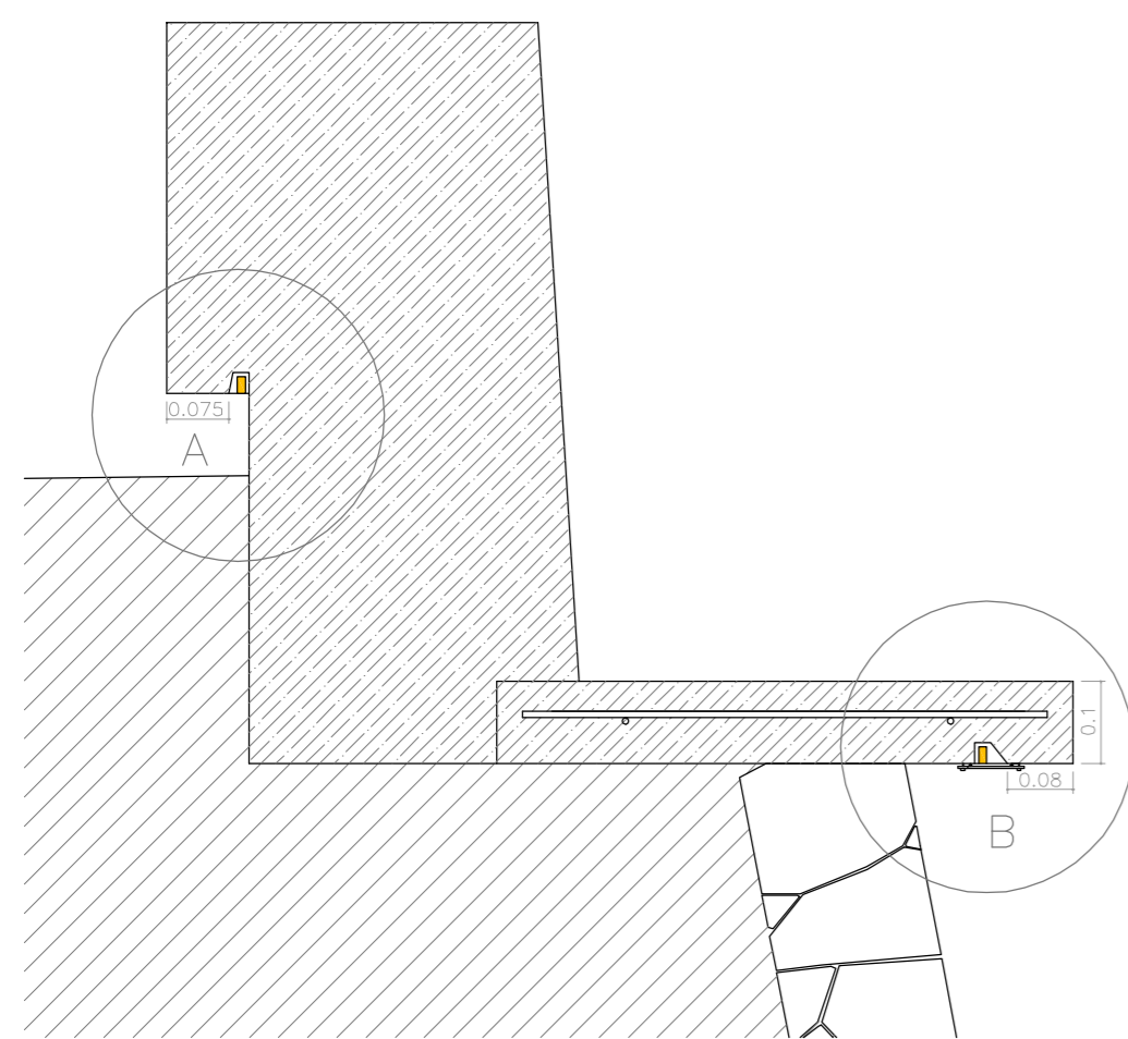
DETALL BANC E. 1/10
